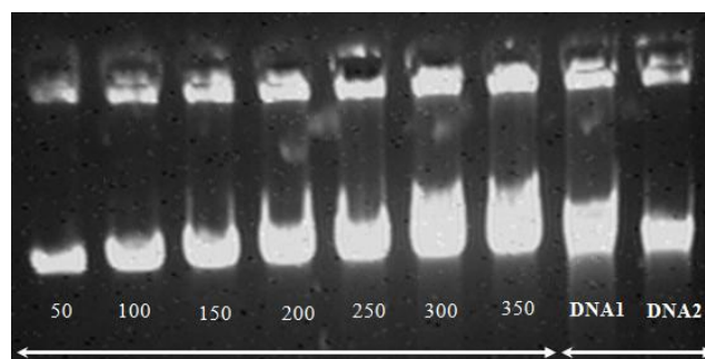
شکل ۱- مقایسه غلظت ۲ نمونه DNA استخراج شده با DNA \lambda
