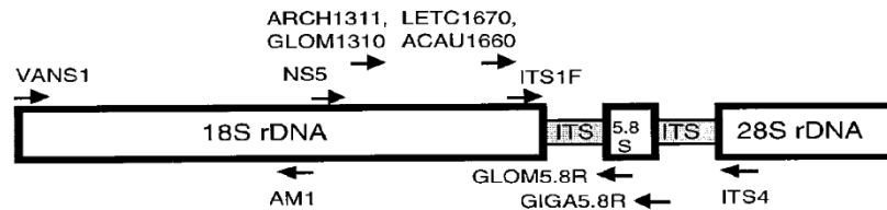
شکل ۲- آغازگرهای اختصاصی طراحی شده توسط Redecker (۲۰۰۰) برای گروه‌های فیلوژنتیک قارچ‌های AM
