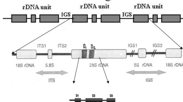
شکل ۱- ژن‌های DNA-ریبوزومی و اجزای سازنده آن (Krishna و Reddy و همکاران ۲۰۰۵)
