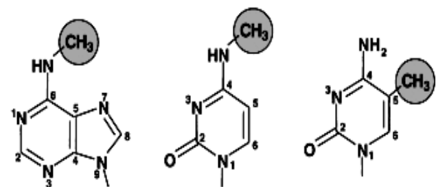
شکل ۲- نمایش ساختار شیمیایی بازهای متیله‌شونده در DNA
