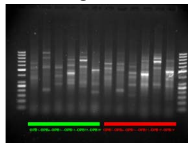
شکل ۲- نمونه از الگوی باندینگ ۶ آغازگر در جمعیت‌های سیاه ماهی C. c. gracilis در ایستگاه‌های بالادست (سمت راست) و پایین دست سد (سمت چپ) شهید رجایی در رودخانه تجن ساری (ژل ۱/۵ درصد آگار)
