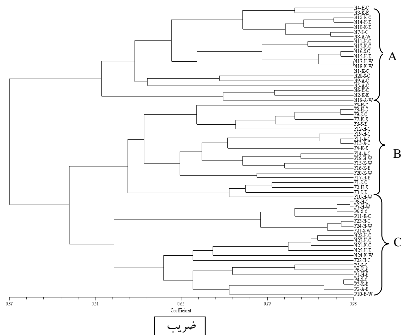
شکل ۲- دندروگرام به دست آمده برای ۶۰ جدایه Xanthomonas oryzae pv. oryzae با استفاده از ضریب تشابه SM و روش UPGMA بر اساس داده‌های RAPD روی DNA ژنومی
