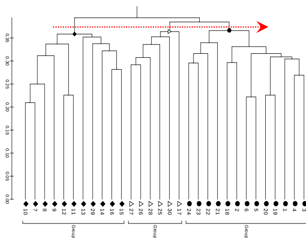
شکل ۳- گروه بندی ۳۰ ژنوتیپ گندم نیای تائوشی، با استفاده از ۶۹ باند نمره‌دهی شده از ۱۷ مکان نشانگرهای ریزماهواره (الگوریتم UPGMA براساس ماتریس عدم تشابه جاکارد).
