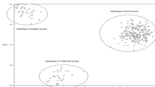
شکل ۲- نمودار پراکنش دو بعدی نژادهای کرد، عرب و ترکمن روی محور مختصات به کمک روش تجزیه به مؤلفه‌های اصلی
