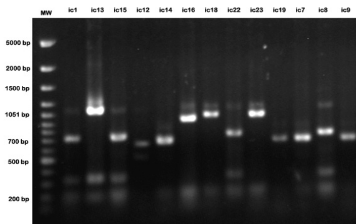
شکل ۳- الگوی هضم ژن 16S rRNA با آنزیم MboI . (از سمت چپ، چاهک شماره ۱) سایز مارکر 100 bp؛ سایر چاهک‌ها الگوی هضم تعدادی از باکتری‌های جداسازی شده (نام جدایه در بالای چاهک آورده شده است).
