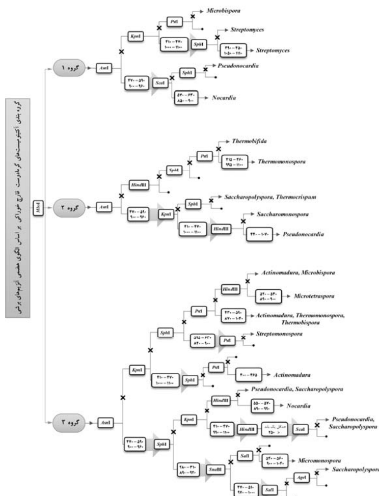
شکل ۴- گروه‌بندی آکتینومیسست‌های گرمادوست قارچ دکمه‌ای براساس الگوی هضمی آنزیم‌های بررسی. جنس‌های هرگروه در پایان مسیر بررسی مشخص شده است. در هر مسیر پس از هضم با آنزیم بررسی ذکر شده در مستطیل، عدم برش با علامت x و باندهای حاصل از هضم در مستطیل نشان داده شده است.
