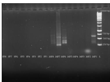
شکل ۲- آزمایش نشانگرهای ریپید A12, K3, OPB01, K4, A10, OPO08, K1 و D10 (P1 to P8) بر روی هر دو توده نر (M) و ماده (F) L: سایز مارکر یک کیلو بازی
