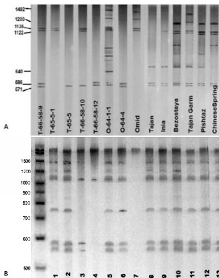
شکل ۵- الگوی بانندی آغازگر S 13 در ارقام و لاین‌های موتانت (A) و ۱۳ نتاج جمعیت F 2 حاصل از تلاقی Tajan×T-66-58-12 (B)
