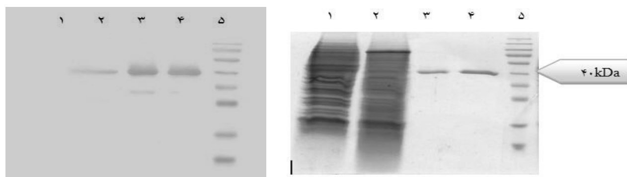
شکل ۶- مطالعه لیپازهای طبیعی و جهش یافته تخلیص شده با ستون کروماتوگرافی تعویض یونی توسط الکتروفورز و وسترن بلات. چاهک ۱) محیط کشت مخمر Gs115 (کنترل منفی)؛ چاهک ۲) محیط کشت بعد از القا؛ چاهک ۳) لیپاز طبیعی خالص (کنترل مثبت)؛ چاهک ۴) لیپاز جهش یافته خالص؛ چاهک ۵) نشانگر وزنی SMO671.
