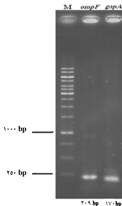
شکل ۱- ژل الکتروفورز محصول PCR. چاهک اول از چپ مربوط به نشانگر DNA و دو چاهک بعدی به ترتیب مربوط به ژن ompF و gapA می باشد. اندازه هر محصول زیر نویس شده است.
