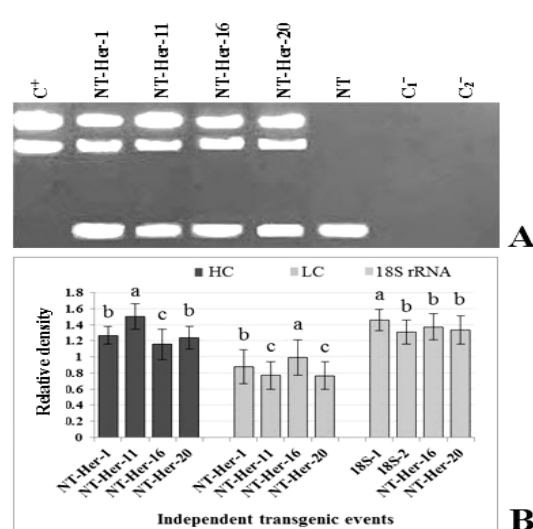
شکل ۶- (A) تجزیه Semi-quantitative RT-PCR در گیاهان توتون تراریخته T_0 حاوی ژن‌های رمز کننده آنتی‌بادی Trastuzumab (A) الکتروفورگرام بیان ژن‌های LC و HC ؛ C_2^+ مخلوط پلاسمیدهای pBIN19-NTopTras-HC, -LC (شاهد مثبت)؛ -16, -11, -20, NT-Her-1) لاین‌های تراریخته توتون T_0 ؛ (NT) گیاه غیرتراریخته (شاهد منفی اول)؛ C_1^- واکنش RT-PCR دارای RNA الگو به صورت بالک از گیاهان تراریخته و تیمار شده با RNase (شاهد منفی دوم)؛ C_2^- واکنش RT-PCR بدون RNA الگو (شاهد منفی سوم). (B) نمودار بیان کمی شده (نسبی) تراژن‌ها بر اساس نرم‌افزار ImageJ 1.47. شدت نوارها پس از نرمال سازی با نوار کنترل داخلی (18S rRNA) مربوط به هر لاین تراریخته به مقدار کمی چگالی تصحیح شده (Adjusted density) تبدیل شدند. مقادیر دارای حروف غیر مشترک بر اساس آزمون LSD از نظر آماری معنی‌دار ( P' < 0.01 ) هستند.
