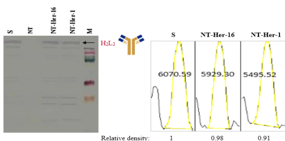
شکل ۷- (A) تجزیه لکه‌گذاری وسترن برای لاین‌های تراریخته توتون T_0 حاوی ژن‌های رمز کننده زنجیره‌های سنگین و سبک Trastuzumab تحت شرایط احیا نشده. (M) نشانگر پروتئینی standard (BioRad)؛ (NT-Her-1 و NT-Her-16) لاین‌های تراریخته مستقل؛ (NT) گیاه غیرتراریخته (شاهد منفی)؛ (S) IgG1 انسانی به عنوان استاندارد. علامت پیکان فرم تترامر (H_2L_2) Trastuzumab به عنوان غالب-ترین فرم تولید شده در گیاهان توتون تراریخته را نشان می‌دهد. (B) پلات پروفیل نوارهای حاصل از الگوی تترامر Trastuzumab. پیک حاصل از هر نوار توسط نرم افزار ImageJ کمی شد و به صورت چگالی نسبی (Relative density) بر اساس نمونه استاندارد بیان شد.
