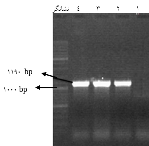
شکل ۳- تایید حضور سازه pEPC در اگروباکتریوم با استفاده از همسانه - PCR با آغازگرهای 35S2fw و Prorv. (چاکک ۱) شاهد؛ چاکک‌های ۲، ۳ و ۴) تکثیر یک قطعه ۱۱۹۰ جفت بازی در همسانه‌های دارای سازه pEPC؛ (نشانگ) GeneRuler DNA Ladder Mix (ف. ممتاز).
