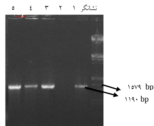
شکل ۲- تایید حضور سازه pLPC در اگروباکتریوم با استفاده از همسانه-PCR با آغازگرهای 35S2fw و Prorv. (نشانهگر) Lambda DNA/ EcoRI HindIII ؛+ چاهک‌های ۱، ۲، ۳، ۵) تکثیر قطعه ۱۵۷۹ جفت بازی در همسانه‌ها، دارای سازه pLPC؛ چاهک ۴) شاهد.
