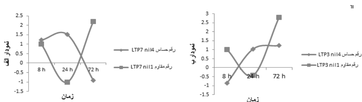
شکل ۶- الگوی بیان ژن LTP در دو رقم حساس Nil4 و مقاوم Nil1 گندم در سه تیمار زمانی ۸، ۲۴ و ۷۲ ساعت پس از آلودگی با بیماری Fusarium graminearum . نمودار (الف) الگوی بیان ژن LTP7 در دو رقم حساس و مقاوم را نشان می‌دهد. نمودار (ب) الگوی بیان ژن LTP3 در دو رقم حساس و مقاوم را نشان می‌دهد.
