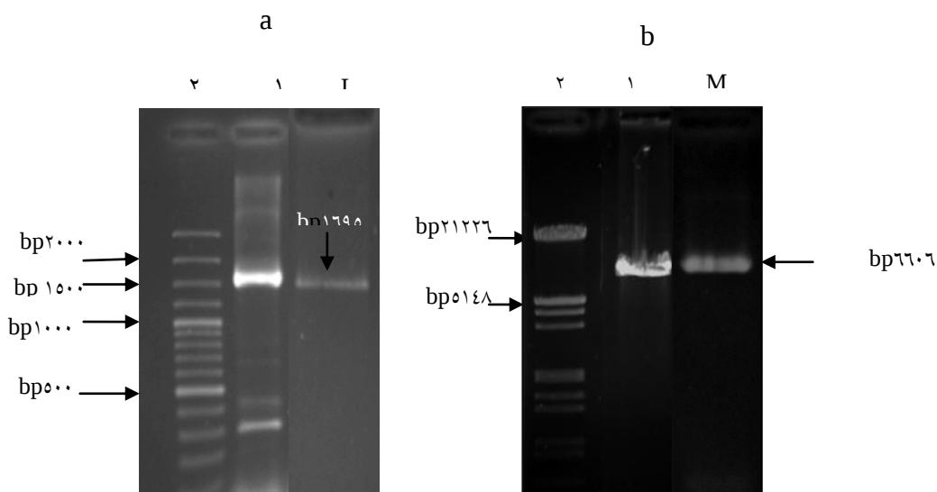
شکل ۴- روند آماده‌سازی ژن LIS و پلاسمید pESC-URA بر روی ژل آگارز. (a) ستون ۱: الکتروفورز محصول PCR ژن LIS ، ستون ۲: خالص‌سازی محصول PCR ژن LIS ؛ (b) ستون ۱: پلاسمید pESC-URA خطی شده با دو آنزیم BamHI و XhoI ، ستون ۲: محصول خالص‌سازی پلاسمید pESC-URA خطی شده از روی ژل، M - نشانگر مولکولی III (فرمنتاس)، (۱۰۰-۳۰۰۰ bp) DNA Ladder؛ L
