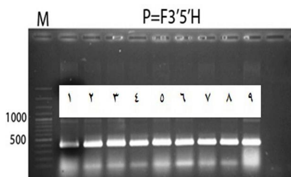
شکل ۵- نتایج تکثیر اختصاصی مکان ژنی P با استفاده از جفت آغازگر P1TaqI در ارقام سیب‌زمینی. ۱. Red Robin ، ۲. Desiree ، ۳. Bildstar ، ۴. Roseval ، ۵. Red Roseval ، ۶. Istanbuli ، ۷. Purple Majesty ، ۸. Picasso ، ۹. Charlotte .
