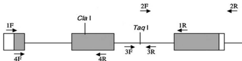
شکل ۴- محل اتصال جفت آغازگرهای اختصاصی P2ClaI-F / P2ClaI-R (4F/4R) و P1TaqI-F / P1TaqI-R (3F/3R) (مشخص شده با پیکان) و محل برش آنزیم‌های TaqI و ClaI در مکان ژنی P .
