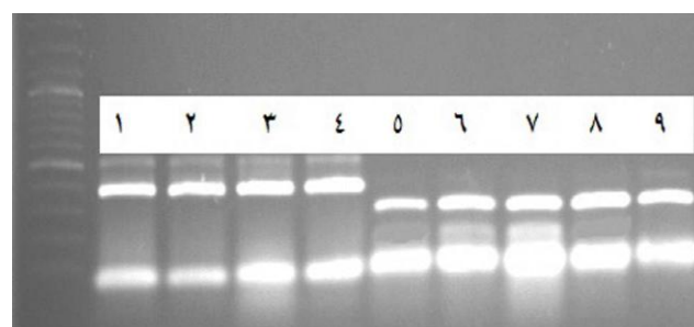
شکل ۶- نتایج هضم آنزیمی با TaqI مکان ژنی P تکثیر شده با جفت آغازگر P1TaqI در ارقام سیب‌زمینی محصول PCR هضم‌نشده (۱) Red Robin ، (۲) Frisia ، (۳) Purple Majesty ، (۴) Picasso و محصول PCR هضم‌شده (۵) Red Robin ، (۶) Purple Pelisse ، (۷) Purple Majesty ، (۸) Bildstar ، (۹) Istanbuli .
