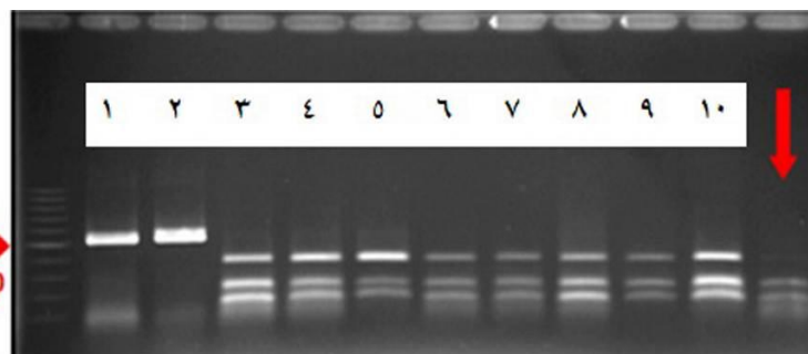
شکل ۹- نتایج هضم آنزیمی با BamHI مکان ژنی P تکثیر شده با جفت آغازگر RBamHI در ارقام سیب‌زمینی.
