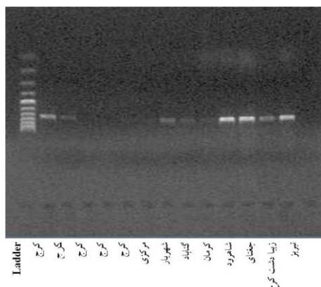
شکل ۱- نمونه‌هایی از تصویر باندهای تشکیل شده بر روی ژل آگارز (سمت راست COI و سمت چپ ITS1)
