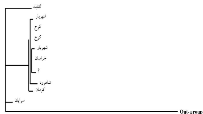
شکل ۵- درخت فیلوژنتیکی به‌دست آمده به‌روش Branch lengths و Linkages برای توالی‌های حاصل از قسمت ITS1
