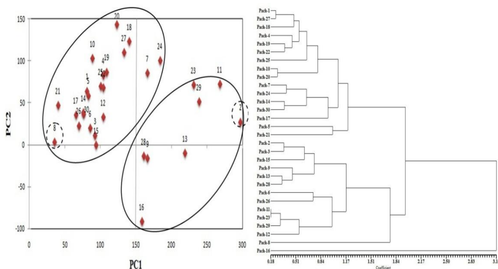
شکل ۱- درخت‌واره حاصل از تجزیه خوشه‌ای دو مؤلفه اصلی داده‌های مورفوژیک و نمودار بای پلات دو مولفه مذکور
