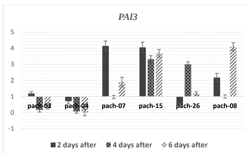
نمودار ۲ - میزان بیان ژن فنیل آلانین آمونیالایز-۳ در ژنوتیپ‌های حساس، متحمل و مقاوم، ۲، ۴ و ۶ روز پس از آلوده‌سازی
