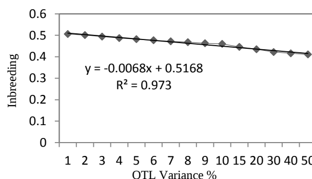
شکل ۲- میزان هم‌خونی ناشی از منظور نمودن مقادیر مختلف واریانس QTL
