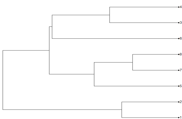
شکل ۴- دندروگرام حاصل از تجزیه کلاستر نمونه‌های مورد بررسی گل محمدی بر اساس داده‌های CBDP با استفاده از ضریب فاصله دایس و روش UPGMA
