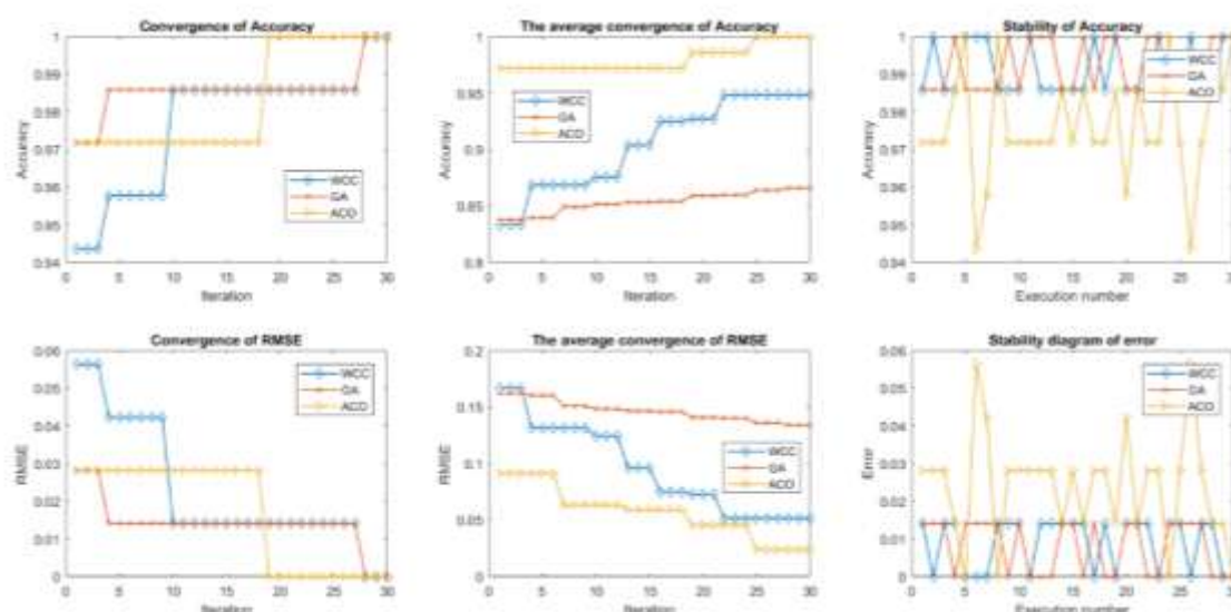
شکل ۶- نمودار همگرایی الگوریتم‌ها
