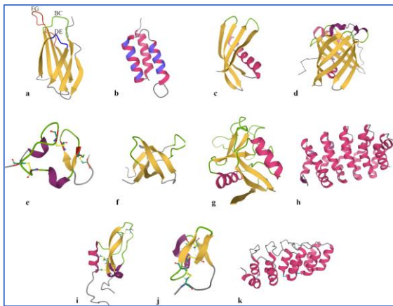
شکل ۱- ساختار سه بعدی مولکول‌های آنتی‌بادی‌نما؛ (a) مولکول ادنکتین (PDB:1TTG)، (b) مولکول افی‌بادی (PDB:1Q2N)، (c) مولکول افیمر (PDB:4N6T)، (d) مولکول آنتی‌کالین (PDB:1LNM)، (e) مولکول اویمر (PDB:1AJJ)، (f) مولکول فینومر (PDB:1M27)، (g) مولکول اتریمر (PDB:1TN3)، (h) مولکول پروتئین تکرار آرمادیلو (PDB:4DB9)، (i) مولکول مهارکننده دمین کونیتز (PDB:2DDI)، (j) مولکول ناتین (PDB:2IT7)، (k) مولکول پروتئین تکرار آنکرین (PDB:4J8Y)؛ نواحی اتصال با رنگ آبی، حلقه‌های متغیر با رنگ سبز و پل‌های دی‌سولفیدی با مدل گوی و میله نشان داده شده‌اند. تصاویر با استفاده از RCSB PDB Mol *Viewer 1.0.1 ایجاد شده‌اند (Sehna et al. 2018).
