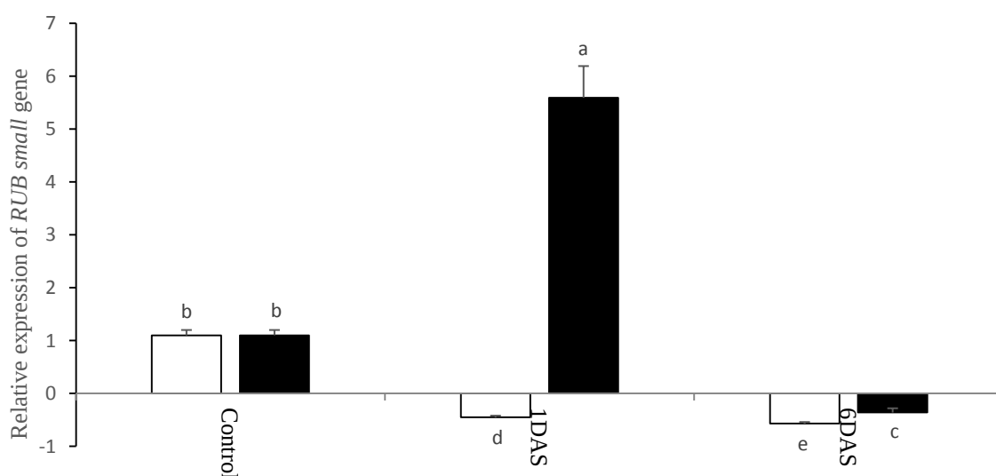
شکل ۳- الگوی تغییر بیان نسبی ژن زیرواحد کوچک روبیسکو ژنوتیپ‌های متحمل Sel96th11439 (ستون سیاه) و حساس ILC533 (ستون سفید) نخود تحت شرایط کنترل، روز اول (1DAS) و روز ششم (6DAS) پس از تنش سرما 4^{\circ}\text{C} .
