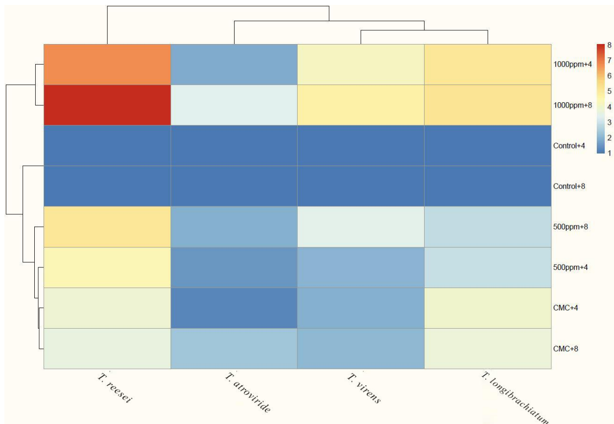
شکل ۲- نمایش نقشه گرمایی سطح بیان ژن Xyl نقشه ارتباط بیان ژن را در چهار گونه قارچ Trichoderma تحت تیمار با سه فاکتور القاگر شامل محیط کشت حاوی CMC، محیط کشت حاوی عصاره جلبکی ۵۰۰ میکروگرم بر میلی‌لیتر و محیط کشت حاوی عصاره جلبکی ۱۰۰۰ میکروگرم بر میلی‌لیتر را نشان می‌دهد. تغییر بیان ژن در گونه‌های دارای دندروگرام‌های مرتبط تشابه بیشتری داشته است. خانه‌های مایل به رنگ آبی سطح بیان ژن پایین‌تر و خانه‌های مایل به رنگ قرمز سطح بیان ژن بالاتری دارند.
