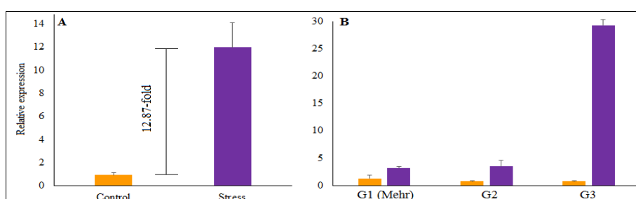
شکل ۱- میزان بیان نسبی ژن SOS1 در دو تیمار عدم تنش و تنش شوری (۲۰۰ میلی‌مولار \text{NaCl} ) (A) و در ژنوتیپ‌های جو (B)
