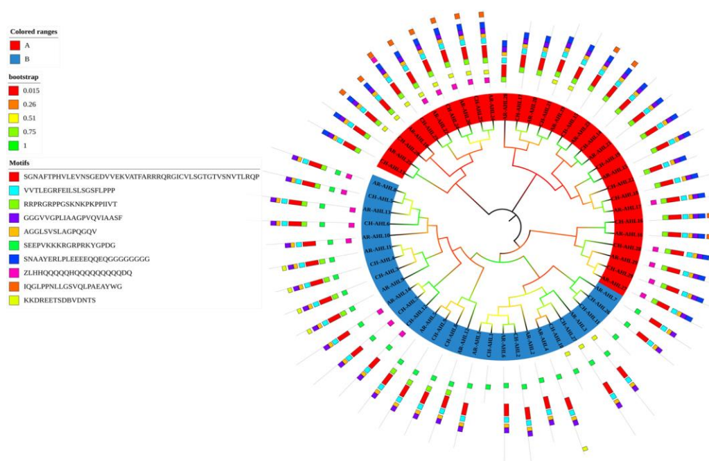
شکل ۲- روابط فیلوژنتیک خانواده ژن‌های AHL با استفاده از MEGA 7 با روش اتصال همسایه (NJ) با ۱۰۰۰ تکرار بوت استرپ ساخته شد. دو کلاسه A و B به صورت دایره رنگی قرمز و آبی به ترتیب نشان داده شد. توزیع موتیف‌های حفاظت شده در پروتئین‌های AHL توسط MEME پیش‌بینی شد. موتیف‌های مختلف با رنگ‌های مختلف ۱-۱۰ نشان داده شد و با برنامه ITOL اضافه شد.
