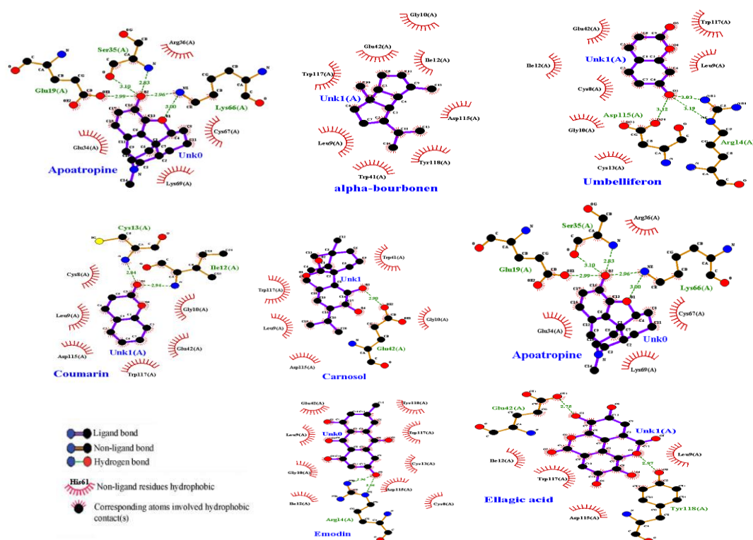
شکل ۲- بررسی اسیدآمینهای درگیر در تشکیل پیوندهای هیدروفوبی و هیدروژنی با استفاده نرم افزار Ligplot+
