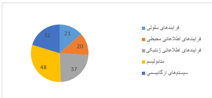
شکل ۴- طبقه‌بندی عملکردی KEGG با استفاده از سرور آنالین KAAS روی ژن‌های هدف پیش‌بینی شده برای میرناهای شناسایی شده در ریواس
