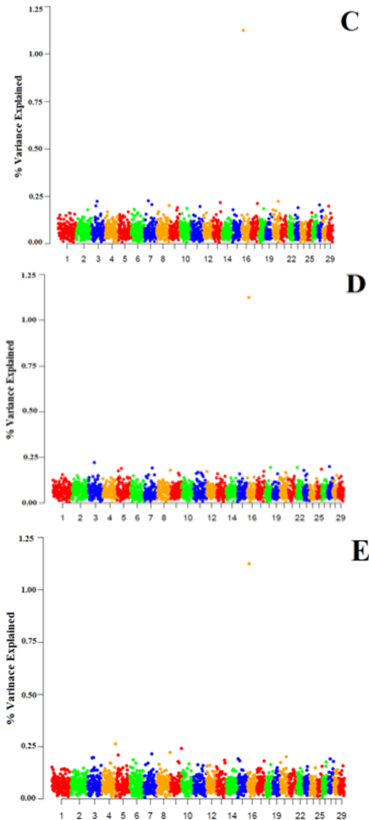
شکل ۱- نمودارهای منحن ارتباط و درصد واریانس ژنتیکی افزایشی توجیه شده حاصل از پنجره‌های ۱ مگابازی مرتبط با (a) طول بدن؛ (b) ارتفاع قد از جدوگاه؛ (c) عمق سینه؛ (d) دور سینه؛ (e) فاصله دو هیپ مبتنی بر روش بیز A.
