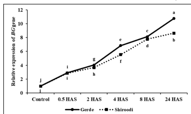
شکل ۳- تغییر الگوی بیان ژن BG در ارقام برنج گرده (خط ممتد) و شیرودی (خط منقطع) در شرایط شاهد و نیم، دو، چهار، هشت و ۲۴ ساعت پس از تنش سرما (HAS). حروف مشابه، عدم اختلاف معنی‌دار را بر اساس آزمون دانکن در سطح یک درصد نمایش می‌دهد.
