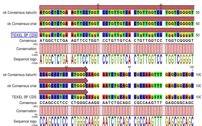
شکل ۳- قسمتی از توالی ژن RNase A هم ردیف شده و ناحیه سیگنال پپتید (پیکان قرمز) از نوکلئوتید ۱ تا ۶۶.
