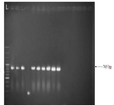
شکل ۲- نتایج حاصل از Colony PCR ژن PAL، چاهک اول Ladder 100bp.
