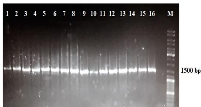
شکل ۲- محصول PCR حاصل از تکثیر ژن 16S rRNA بر روی ژل آگارز. ۱) سویه Sav1، ۲) سویه Sav1S، ۳) سویه Sav42، ۴) سویه Tal21، ۵) سویه Tal22، ۶) سویه Tal31، ۷) سویه Tal32، ۸) سویه Tal41، ۹) سویه Tal42، ۱۰) سویه Tal51، ۱۱) سویه Tal52، ۱۲) سویه Tal6، ۱۳) سویه Tal62، ۱۴) سویه Tal71، ۱۵) سویه Tal72، ۱۶) سویه Krj1
