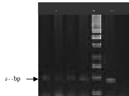
شکل ۷: آنالیز گیاهان تراریخت با استفاده از PCR و آغازگرهای اختصاصی IFN \gamma ؛ خط ۱، ۲، ۳، ۴: گیاهان تراریخت شده، خط ۵: نشانگر وزنی ۱ kb، خط ۶: کنترل مثبت (پلاسمید pBI121 حاوی سازه)؛ خط ۷: کنترل منفی (گیاه غیرتراریخت)
