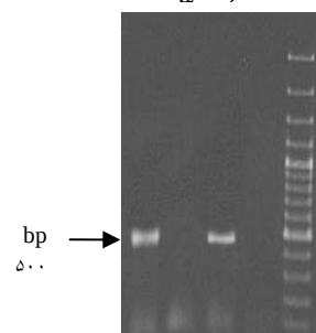
شکل ۸: آنالیز گیاهان تراریخت با RT-PCR و آغازگرهای اختصاصی IFN \gamma ؛ خط ۱: کنترل مثبت (پلاسمید pBI121 حاوی سازه ترکیبی)؛ خط ۲ و ۳: گیاهان تراریخت، خط ۴: کنترل منفی (گیاه غیرتراریخت)، خط ۵: نشانگر ۱۰۰bp
