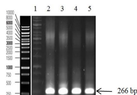
شکل ۴- محصول Gradient-PCR قطعه سنس از ژن امگا گلیادین از DNA ژنومی. ۱- نشانگر وزنی مولکولی (۱ kb DNA - شرکت فرمنتاز) ۲، ۳، ۴، ۵- محصول PCR در دماهای ۶۰، ۶۲/۶، ۶۵/۳ و ۶۸ درجه سانتی‌گراد.
