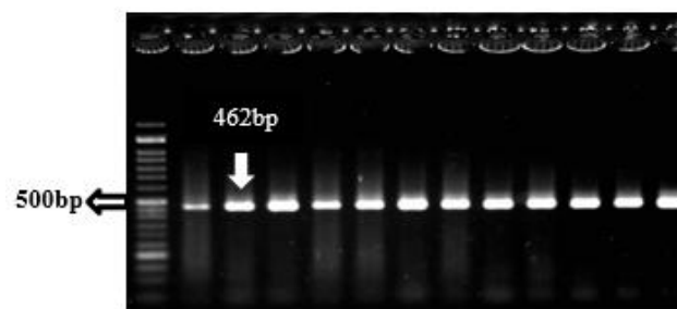
شکل ۱- محصولات PCR حاصل از تکثیر قطعه ۴۶۲ جفت‌بازی از آگرون یک ژن GDF9 (Marker Ladder 50 bp)
