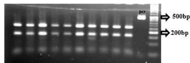
شکل ۲- ژنوتیپ GG مشاهده شده حاصل از هضم آنزیمی قطعه ۴۶۲ جفت
