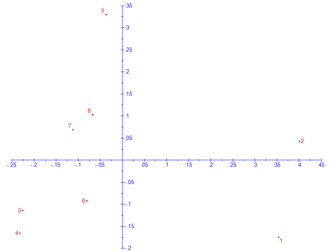
شکل ۶- نمودار بای پلات حاصل از تجزیه به مختصات اصلی (PCoA) برای ۸ نمونه گل محمدی بر اساس داده‌های CDBP
