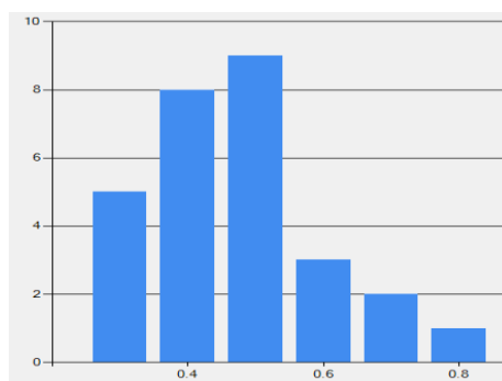
شکل ۲- توزیع فراوانی فواصل ژنتیکی برآورد شده بین جفت نمونه‌های مورد بررسی
