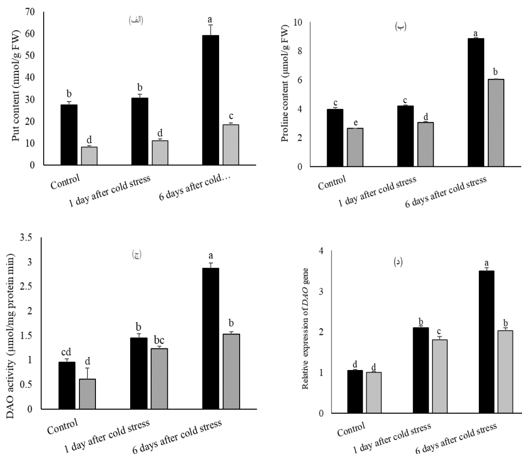
شکل ۳- تغییر میزان پوتری سین (Put) (الف) و پرولین (ب)، فعالیت آنزیم دی‌آمین‌اکسیداز (DAO) (ج) و بیان ژن دی‌آمین‌اکسیداز (DAO) (د) در ژنوتیپ‌های متحمل Sel96th11439 (ستون سیاه) و حساس ILC533 (ستون خاکستری) نخود تحت تیمارهای دمایی شامل دمای طبیعی ( 23^{\circ}C )، روز اول و روز ششم تنش سرما ( 4^{\circ}C ). حروف متفاوت نشان دهنده اختلاف معنی‌دار بین میانگین‌ها براساس مقایسه میانگین دانکن.
