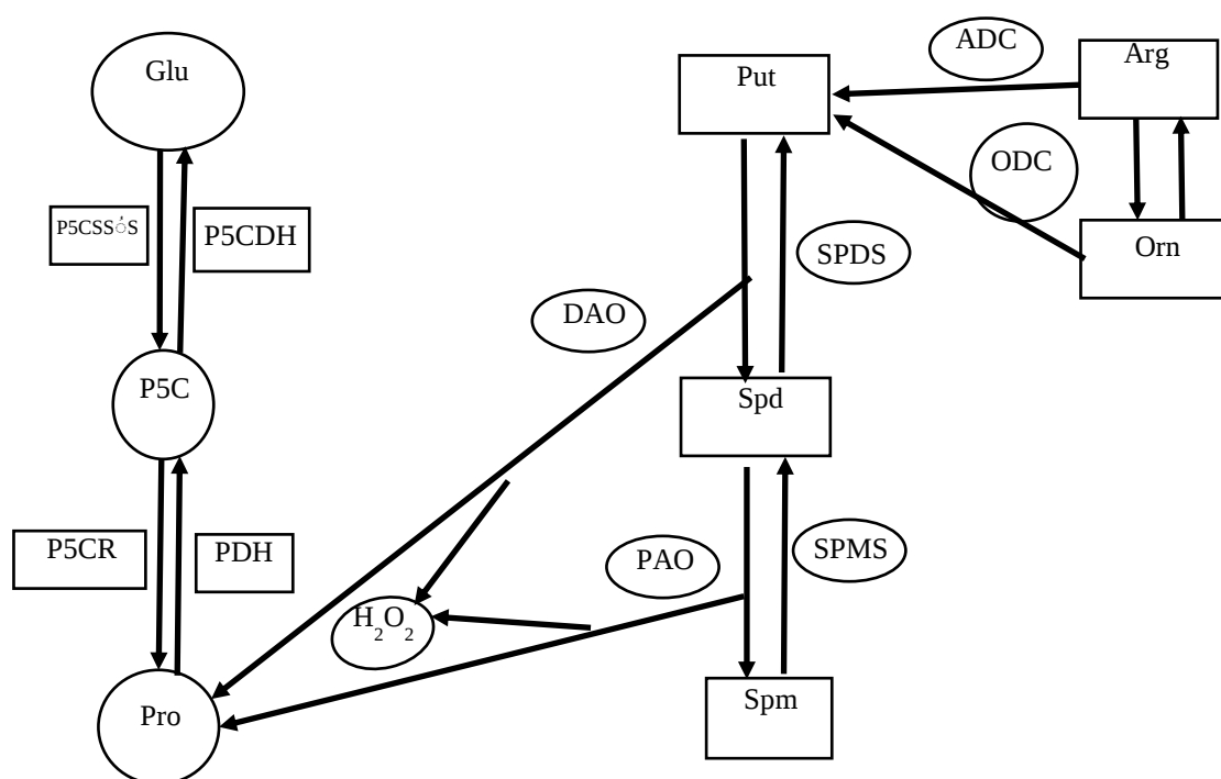
شکل ۱- نمایش شماتیک مسیر پیوستن یولین در گیاهان
