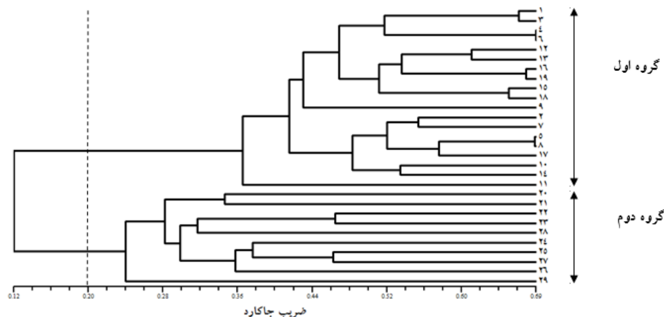
شکل ۲- دندروگرام حاصل از تجزیه خوشه‌ای بر اساس ضریب تشابه چاکارد و روش UPGMA با استفاده از نشانگر ISSR (شماره‌ها بیانگر اکسشن‌ها طبق جدول ۱ می‌باشند).
