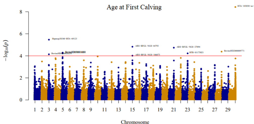
شکل ۲- نمودار منهن صفت سن در اولین زایش، محور X مکان نشانگرها روی کروموزوم، محور Y منفی لگاریتم بر مبنای ۱۰ معیار Pvalues و خط قرمز رنگ نشانه آستانه معنی داری 10^{-4} می باشد.
