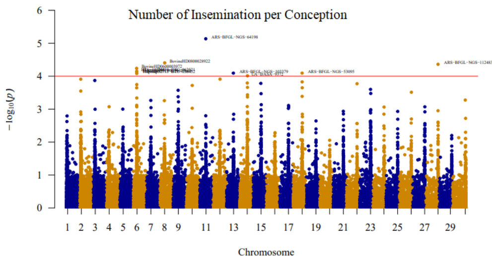
شکل ۳- نمودار منهن صفت تعداد تلقیح به ازای آبستنی محور X مکان نشانگرها روی کروموزوم، محور Y منفی لگاریتم بر مبنای ۱۰ معیار Pvalues و خط قرمز رنگ نشانه آستانه معنی داری 10^{-4} می باشد.
